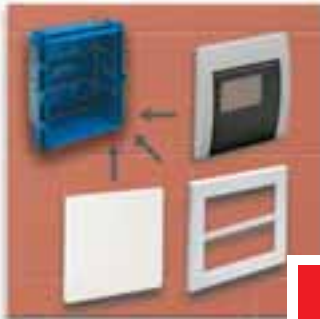
PARETI TRADIZIONALI (FORATO ROSSO) TRADITIONAL WALLS (RED BRICKS)
