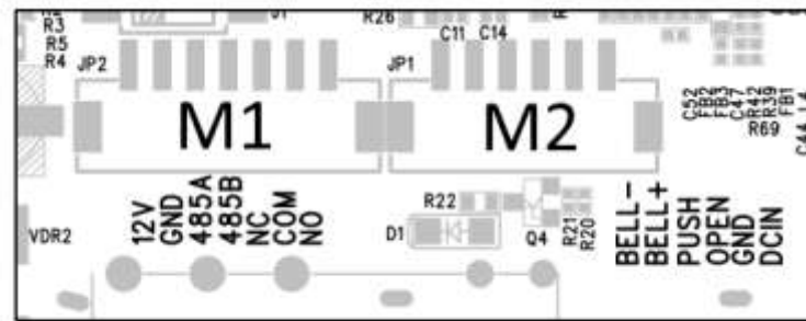
Figura 2.3 Morsettiera
