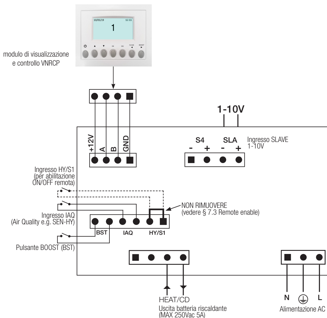
Fig. 5.g Collegamenti elettrici sulla scheda madre fissata all'interno della scatola portacontatti
