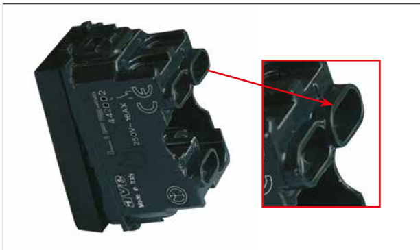
Morsetto "comune" rialzato per un'immediata individuazione "Common" terminal raised for immediate identification
