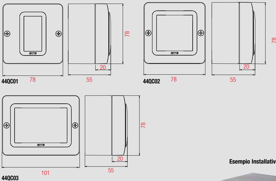
Dimensioni d'ingombro (in mm) Dimensions (mm)
