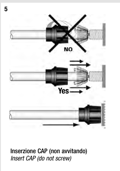
Inserzione conduttore centrale su connettore F femmina Insert central conductor on F-type female connector
