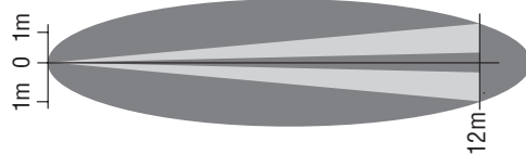
Vista laterale con parzializzatore lente
