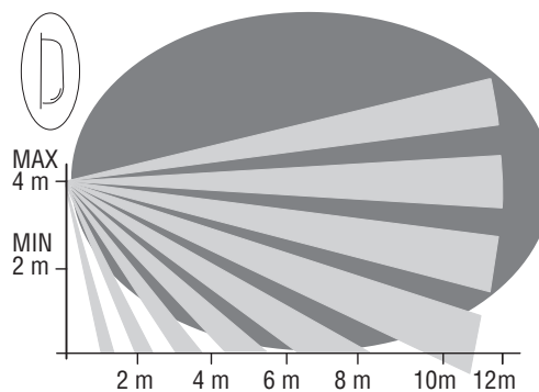
Vista laterale
