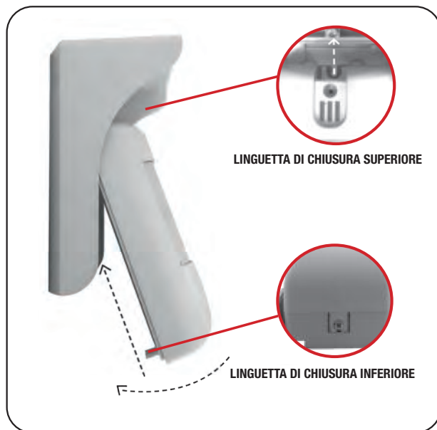
Vista laterale
