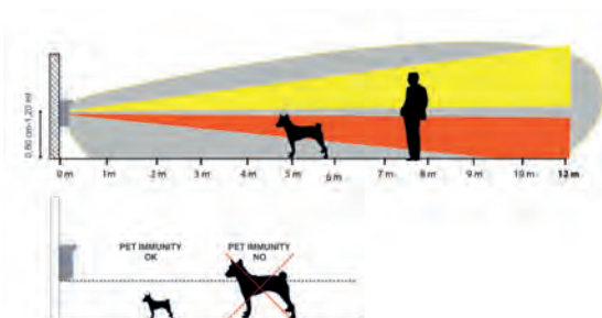
Altezza installazione
