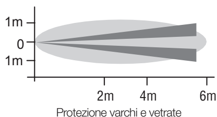
Vista dall'alto
