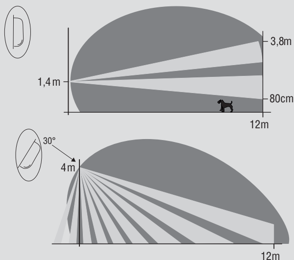
Vista laterale con parzializzatore lente - Side view with blinding lens
