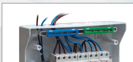
Predisposizione fissaggio morsettiere Predisposition for terminal fixing
