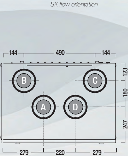
Vista dall'alto View from above
