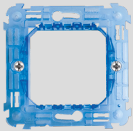
44A02VT 1-2 modules frame for round or square box - with screws إطار لعلبة تركيب مستديرة أو مربعة-مع براغي - وحدة 1- أو 2 S44
