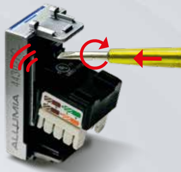
Sgancio Uncoupling
