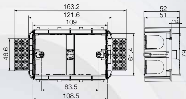
Dimensioni d'ingombro Mounting dimensions
