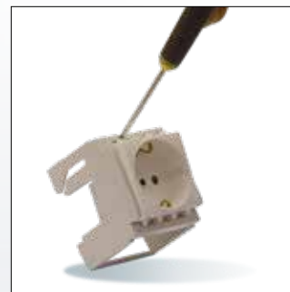
Rimozione frontale dei frutti, semplice e veloce Easy and simple frontal removal of devices
